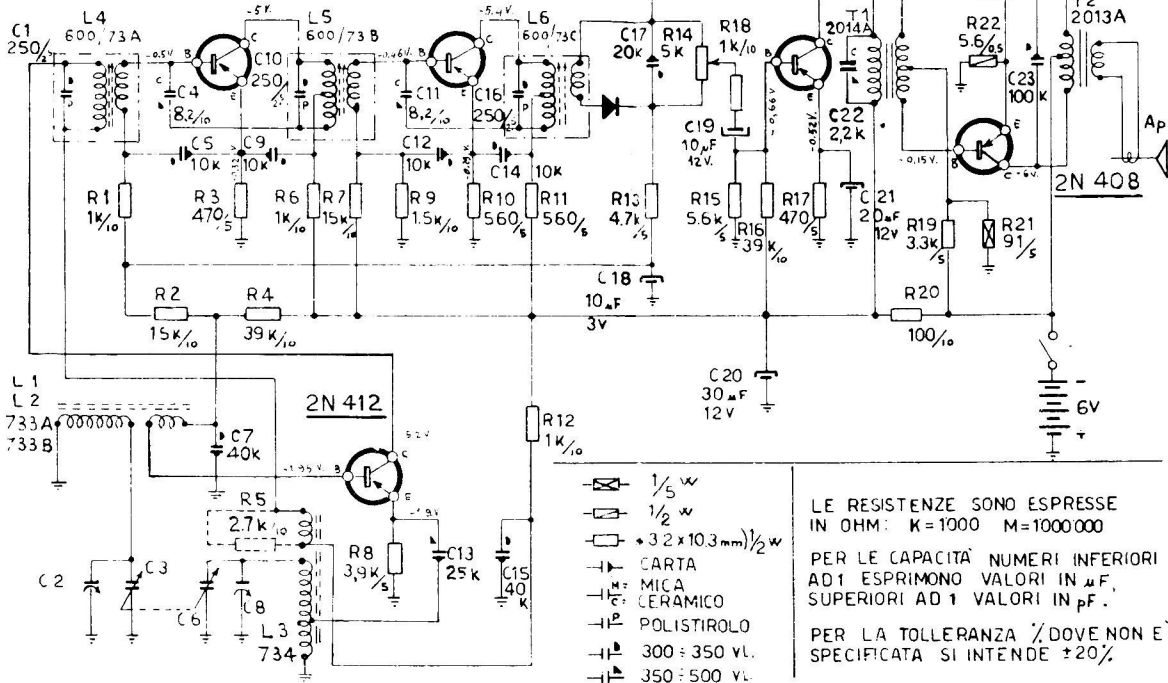
RADORICEVITORE A 6 TRANSISTORI - Mod. S 2011 della « ALLOCCHIO-BACCHINI ».
