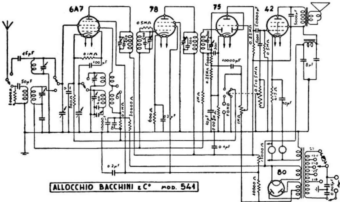
ALLOCCIO, BACCHINI e Co. — Mod. 541 e 541 R. — Produzione 1937-38. — Media frequenza: 425 kHz.
