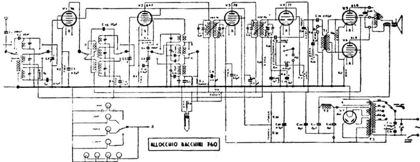
ALLOCCIO, BACCHINI e Co — Mod 760 M 760 R e 760 G — Produzione 1938-39 — Media frequenza: 425 kHz.
