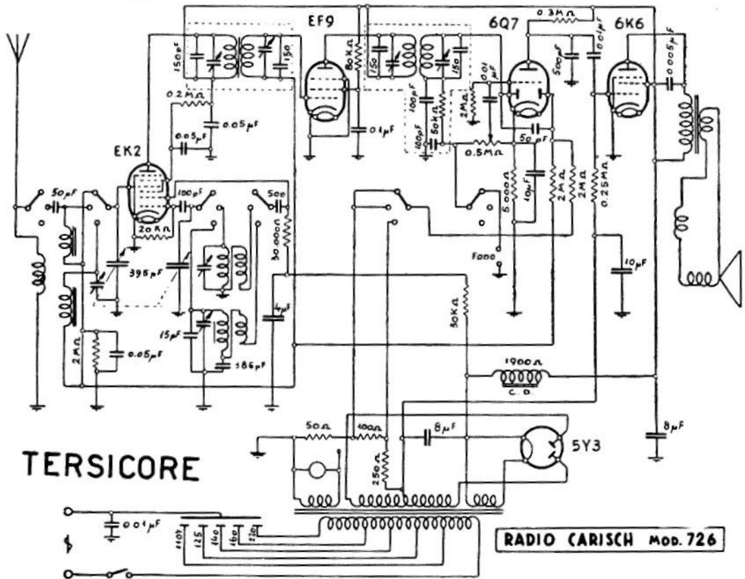
RADIO CARISCH. — Mod. « Tersicore ». — Dall'apparecchio n° 1 al n° 1008 (v. lo schema « Veneto » per i numeri dal 1009 in avanti). — Produzione 1938-1939. — Media frequenza: 485 kHz.
