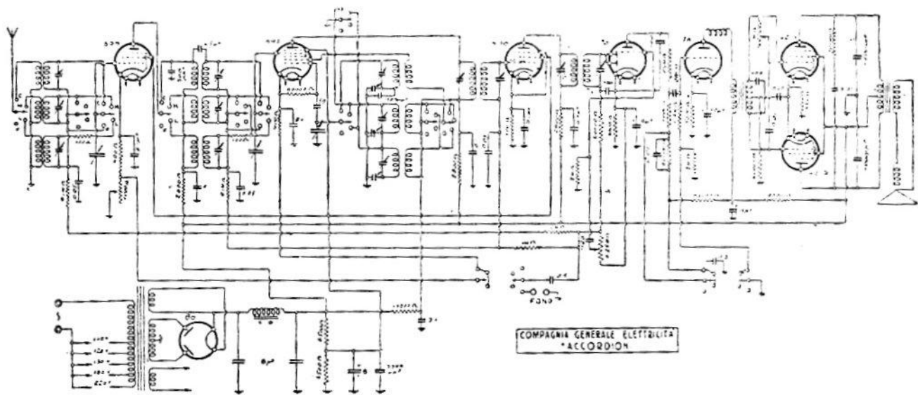
COMPAGNIA GENERALE DI ELETTRICITA — Modello « Accordion ». — Produzione 1936 Media frequenza: 460 kc.
