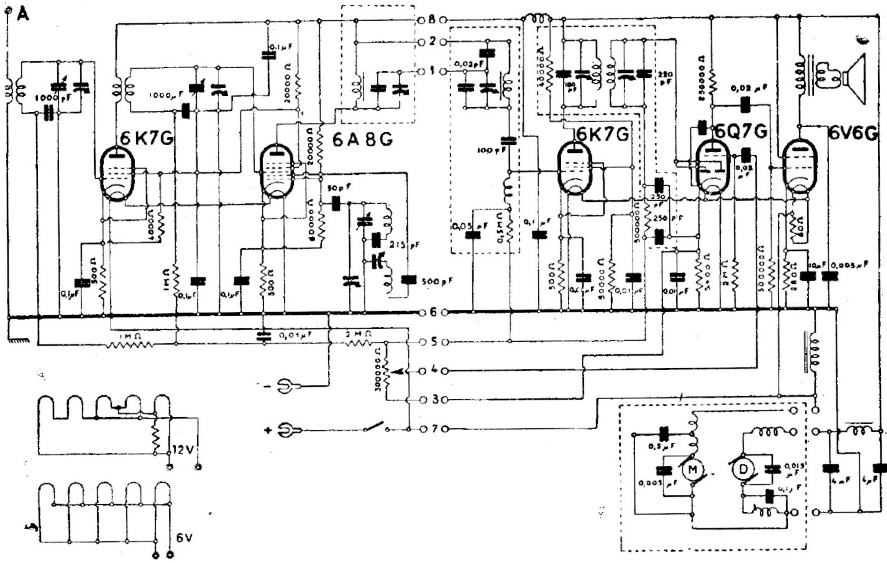
COMPAGNIA GENERALE DI ELETTRICITA' . MOD. «AUTORADIO 61»
