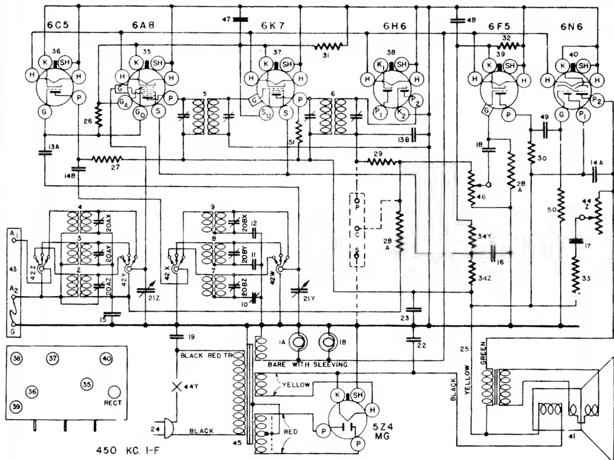
WIRING DIAGRAM—MODEL 716
