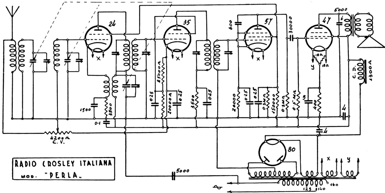
Onde medie. - M. F. 175 kc. - C. V. - 24 oscillatrice-modulatrice. - Produzione 1933. - Potenza d'uscita: 2,5 watt.
