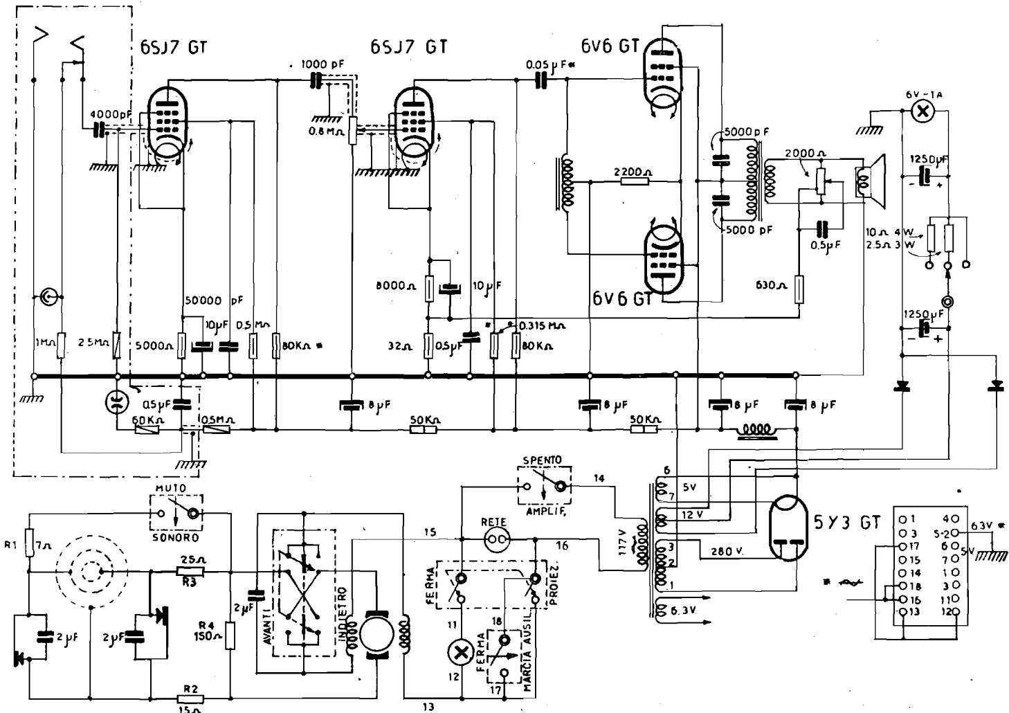
DUCATI - Impianto cinesonoro mod. Club. Per film a passo ridotto. Potenza 8 watt, con 3% di armoniche. Risposta di frequenza da 50 a 7000 cicli. Presa per rivelatore o microfono. Controllo di responso a reazione inversa.
