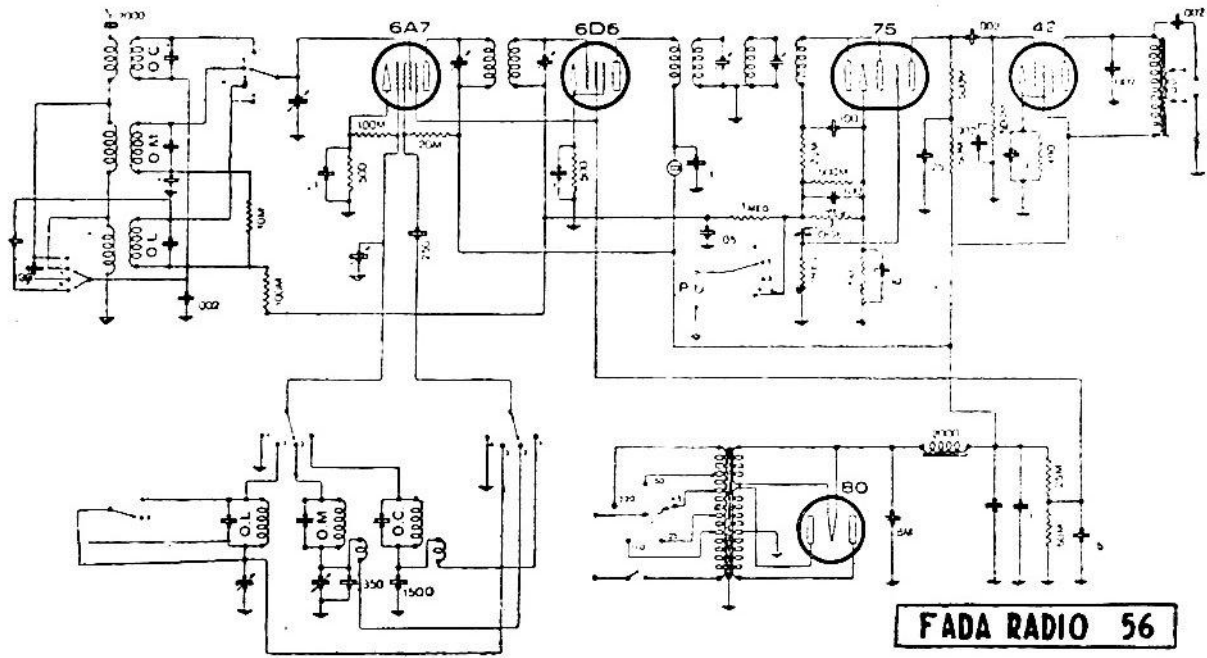
FADA RADIO. - La Precisa. - Mod. 56 (551-552). - Produzione 1937. - Media frequenza: 470 kHz.
