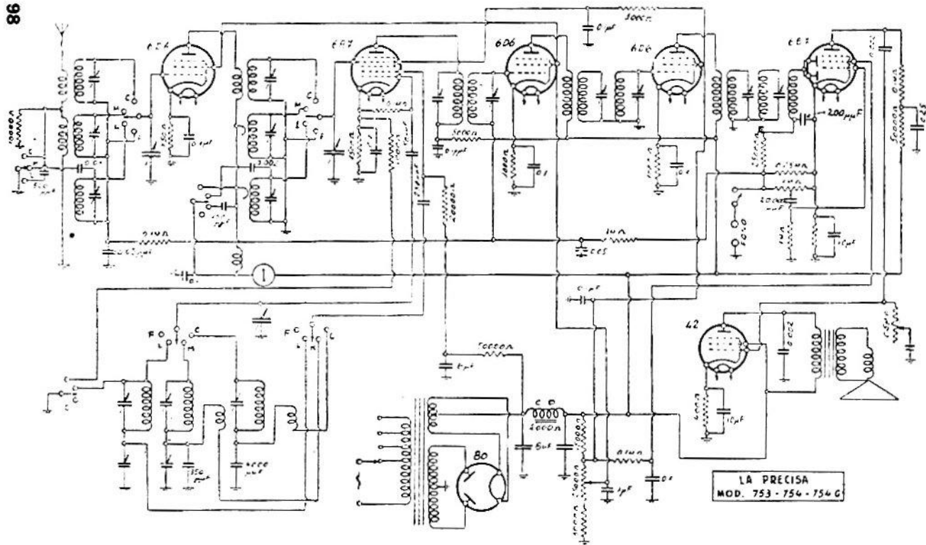
La Precisa. - FADA RADIO - Modelli: « 753, 754 e 754 G ». - Produzione 1935 - Medio frequenza: 470 kc
