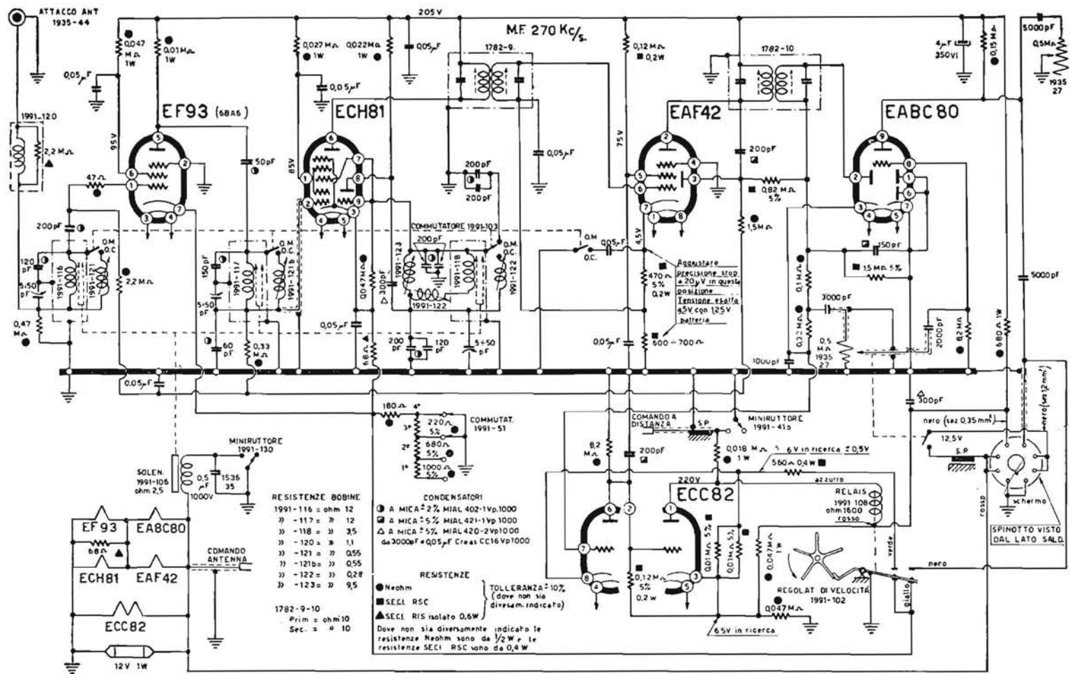
GALLO-CONDOR - Sintonizzatore per autoradio mod. S9-II serie A. Sintonia a permeabilità variabile. Gamme d'onda medie e corte. Ricerca automatica delle emittenti e dispositivo per il comando a distanza. Media frequenza 470 kc/s. Stadio finale e alimentatore v. schema a parte.
