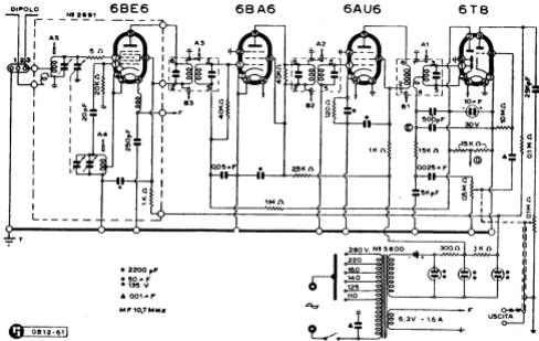
GELOSO S.A. - Sintonizzatore Mod. G 430 FM
