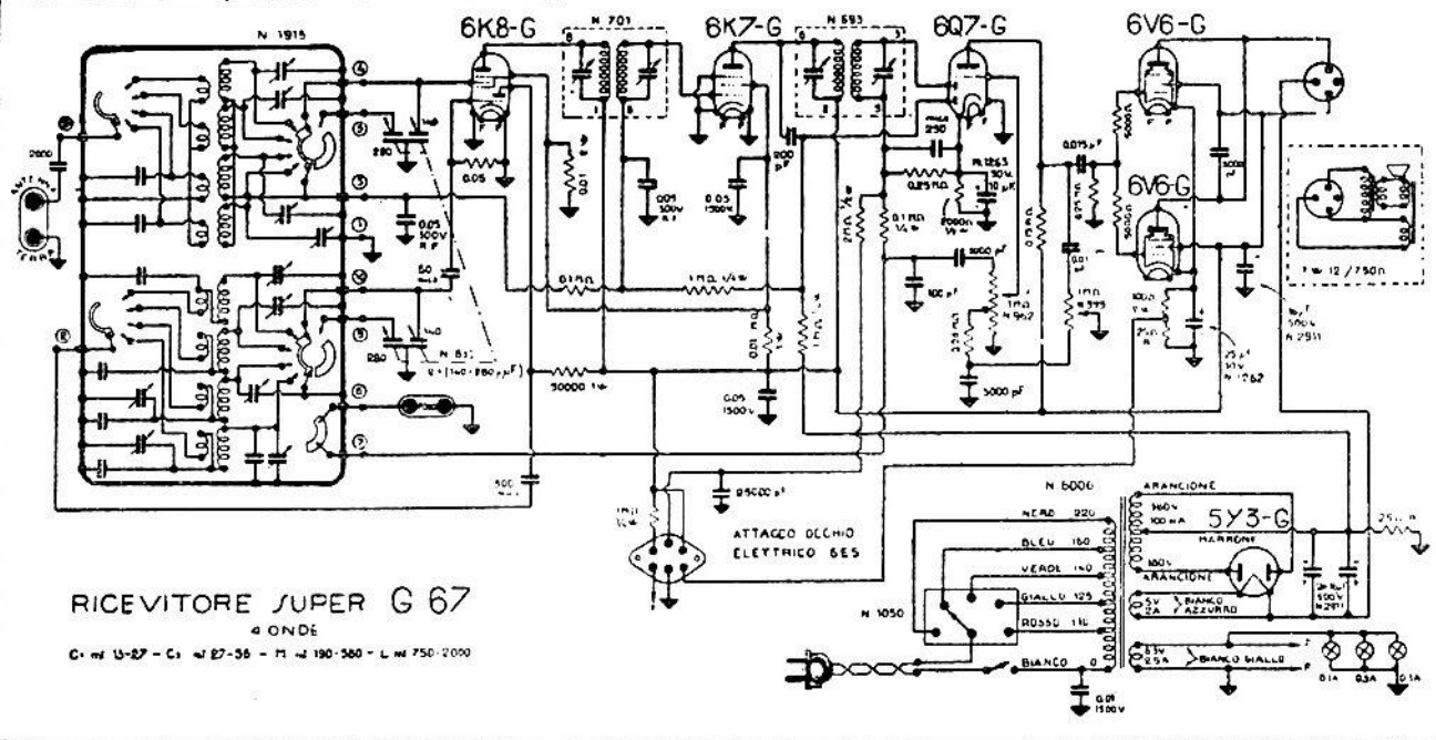
S. A. GELOSO. — Mod. G. 67. — Super a 4 gamme. — Media frequenza: 467 kHz. — Produzione 1939.
