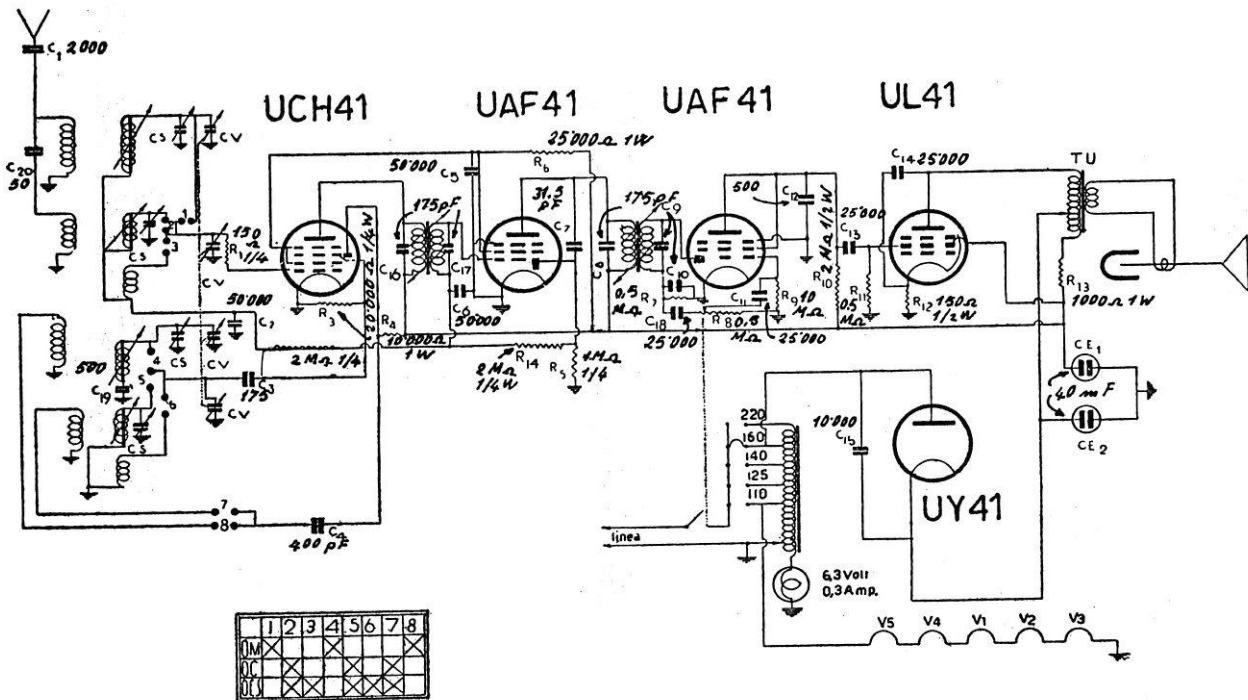
INVAR - Mod. VZ 507-508 - Onde medie e due corte. Potenza d'uscita 2 watt. Consumo 45 watt.
