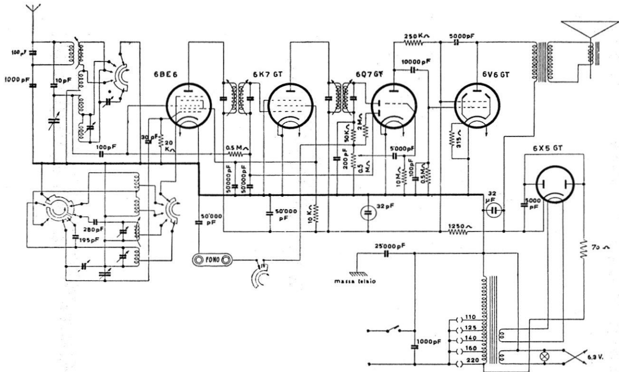
IRRADIO - Mod. AK 14 e AK 15 - Media frequenza 467 kc. Potenza d'uscita 3 watt. Consumo 40 watt.
