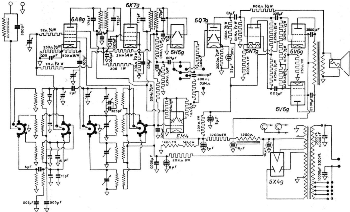
IRRADIO - Mod. DZ 824 - Gamme come modello EX 25. Due 6V6 G finali in controfase, precedute da una 6N7 amplif. BF e invertitrice di fase. Potenza d'uscita circa 12 watt. Ohm eccitazione: 1200. Media frequenza: 450 kc/s. Produzione 1945-46.
