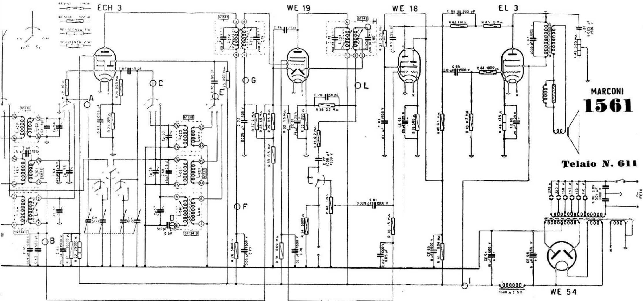
-A VOCE DEL PADRONE. — Mod. « Marconi 1561 ». — Serie sintorapida. — Le valvole indicate nello schema possono venir sostituite come segue: BCH3 senza sostituzione: WE19 con EBF2, WE18 con EFM1, EL3 con WE54. — Potenza d'uscita ca. 3 watt. — Media frequenza; 465 kHz.
