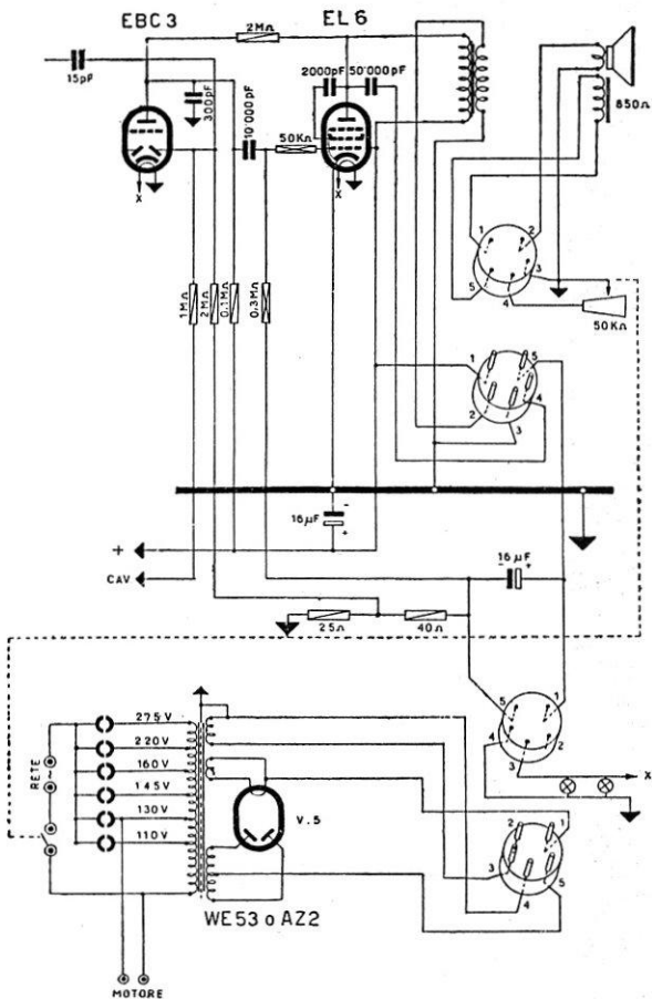
VOCE DEL PADRONE - Mod. 1708 - Del tutto eguale al mod. 1706, dal quale differisce per avere l'indicatrice di sintonia EM4. scritta nel capitolo VII. Media frequenza 465 kc.
