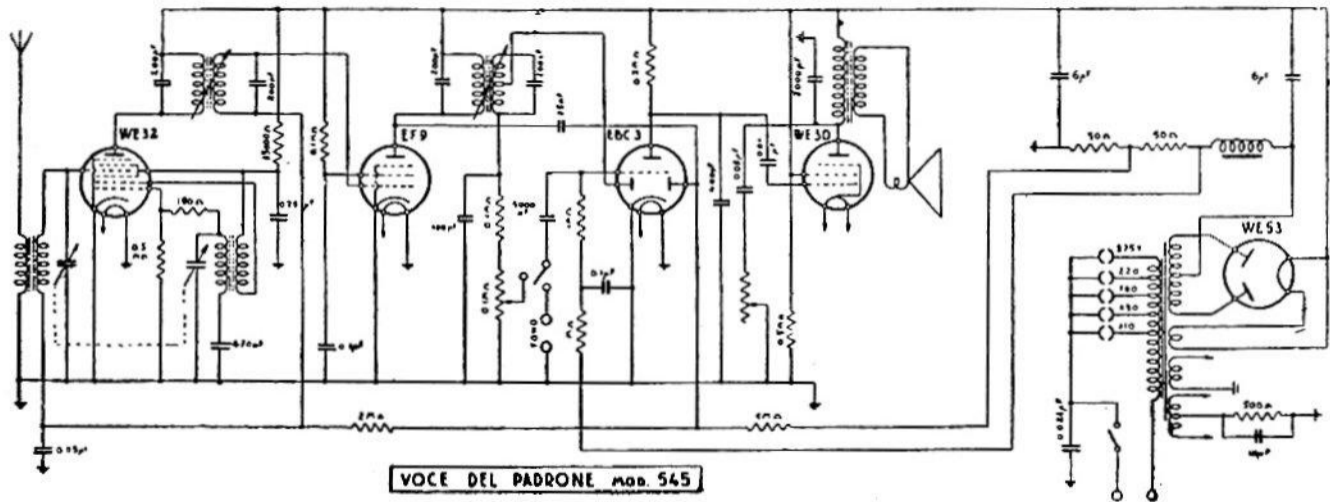
LA VOCE DEL PADRONE — Mod. 545. — Produzione 1938-39. — Media frequenza: 465 kHz.
