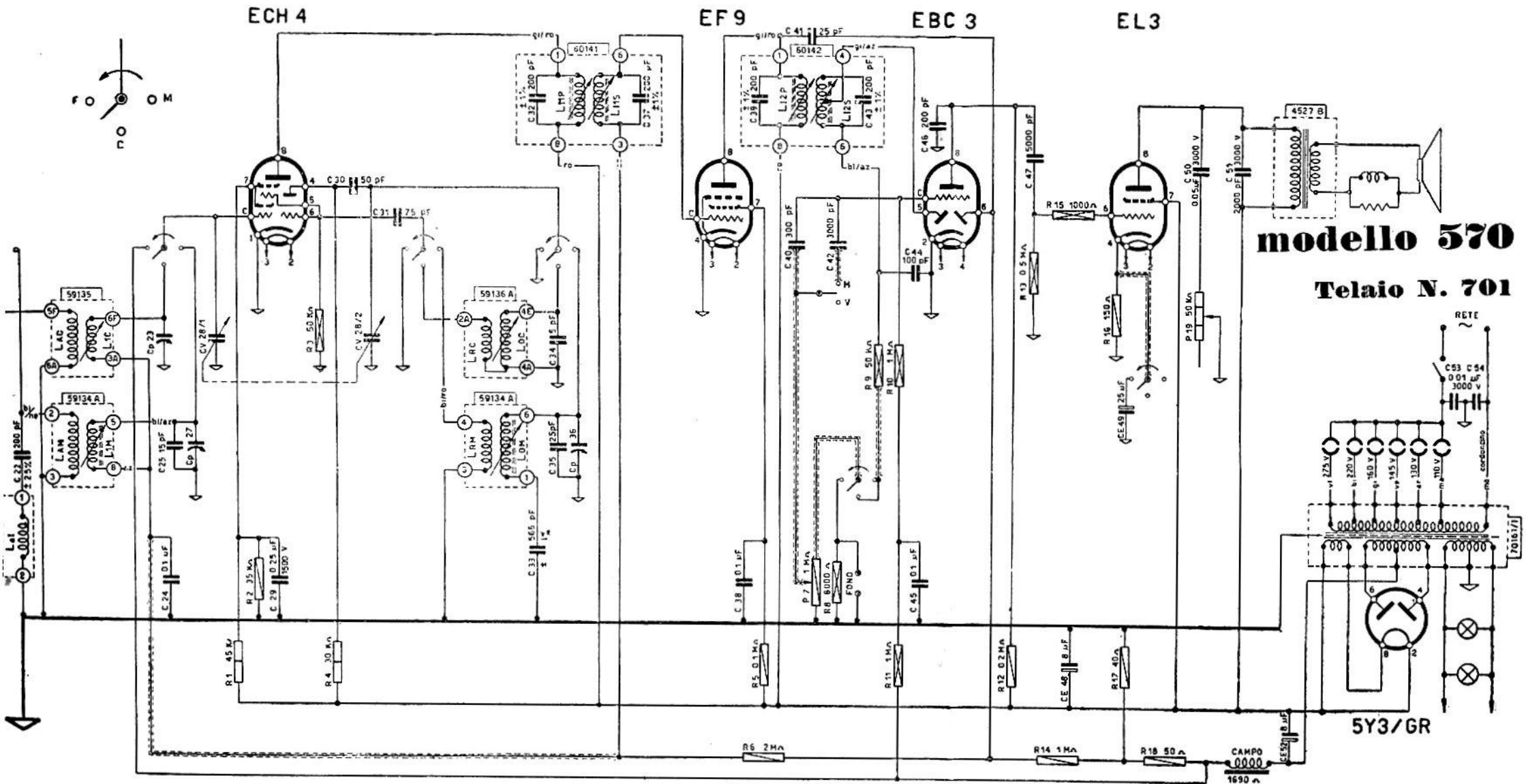
LA VOCE DEL PADRONE. — Mod. 570. — Telaio 701. — Serie sintorapida. — Produzione 1941-1942. — Due gamme d'onda; onde medie 190 a 580 m; onde corte e cortissime 14,5 a 52 m. — Media frequenza: 465 kHz.
