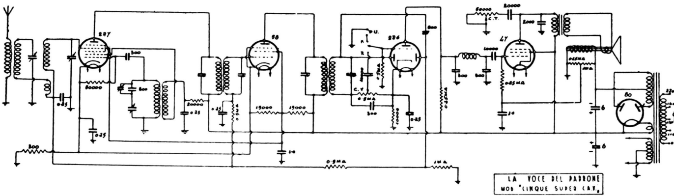
Onde medie. - M. F. 175 kc. - C. A. V. - C. T. - 2A7 oscill.-demod. con accoppiamento elettronico; 58 amplif. m. f.; 2A6 demodul. - c.a.v.; 47 finale di potenza. - Produzione 1934. - Potenza d'uscita: 2,5 watt.
