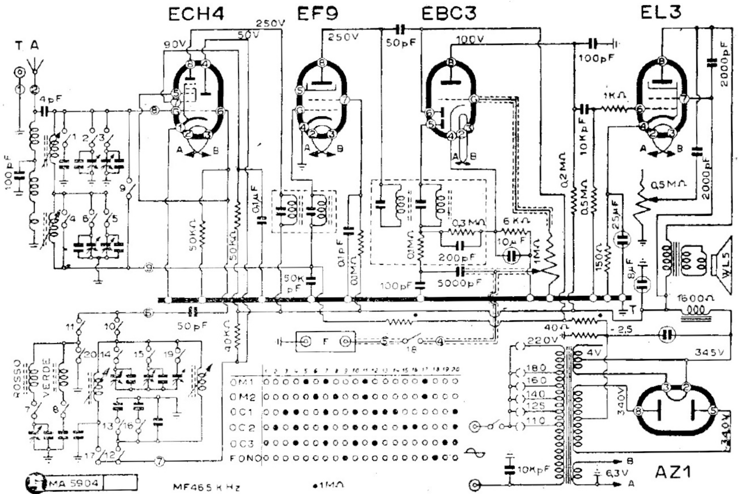
L.I.A.R. - MODD. « 555 » « 555-B »
