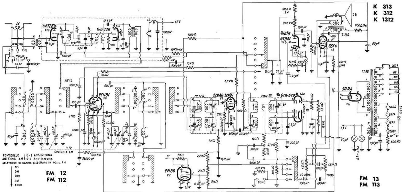
MAGNADYNE RADIO - Modd. FM 12, FM 13, FM-112 e FM 113, K 312, K 313 e K 1312. Apparecchio a modulazione d'ampiezza e di frequenza, con gamma onde medie, due gamme onde corte e una banda onde ultracorte a modulazione di frequenza. Media frequenza AM a 471 kc/s, FM a 10,7 Mc/s. Potenza d'uscita 4 watt.
