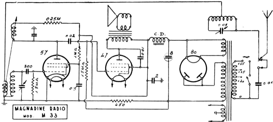
Rivelatrice in reazione (57) seguita dalla finale di potenza (47). - Filtro d'antenna. - Diffusore dinamico. Potenza d'uscita: 1,5 watt.
