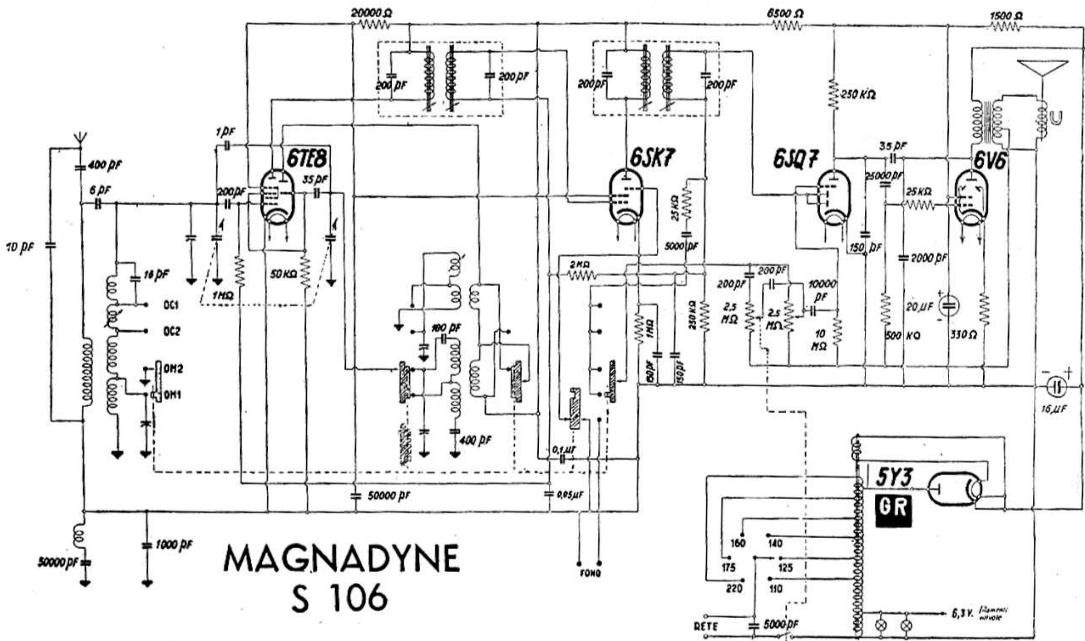
MAGNADYNE RADIO - Mod. MAGNADYNE S 106, mod. DAMAITER M 906, e mod. KENNEDY K 390 - Gamma onde medie divisa e due gamme onde corte. Media frequenza 471,5 kc. Potenza d'uscita 3 watt.
