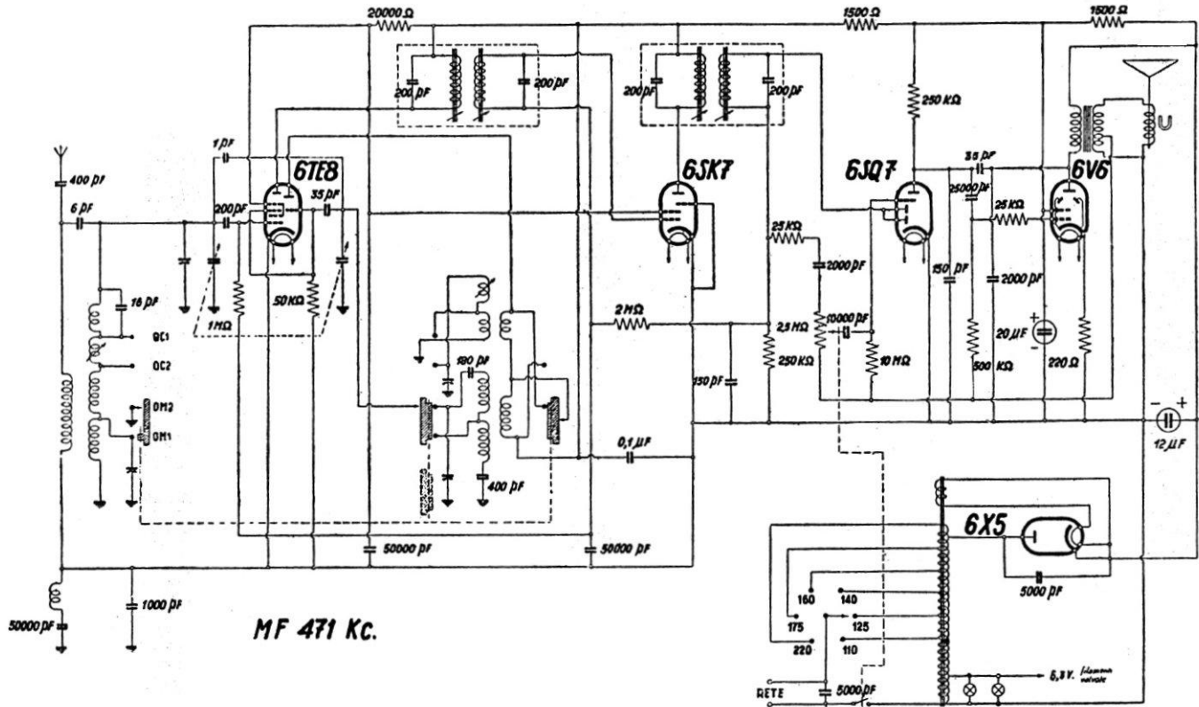
MAGNADYNE RADIO - Modd. S 22, S 23, S 24, S 32 e S 34 - Gamme medie e corte divise. Media frequenza 471 kc. Uscita 3 watt.
