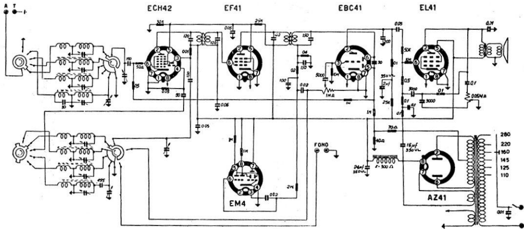
MINERVA RADIO - Mod. 505/4 - Medie e due corte. Media frequenza 470 kc. Particolare tipo di reazione inversa.
