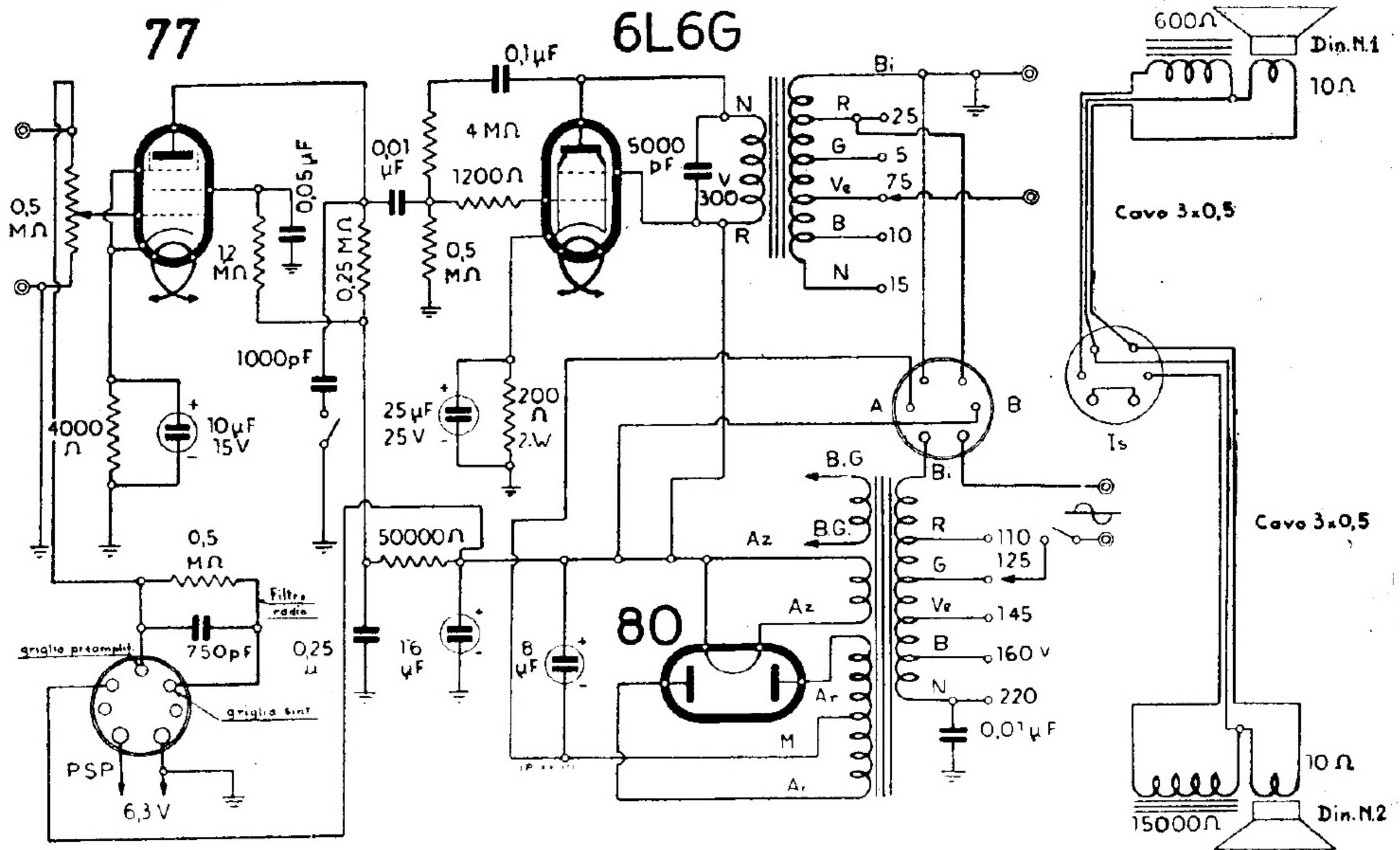
NOVA - AMPLIFICATORE MOD. « 10 W »
