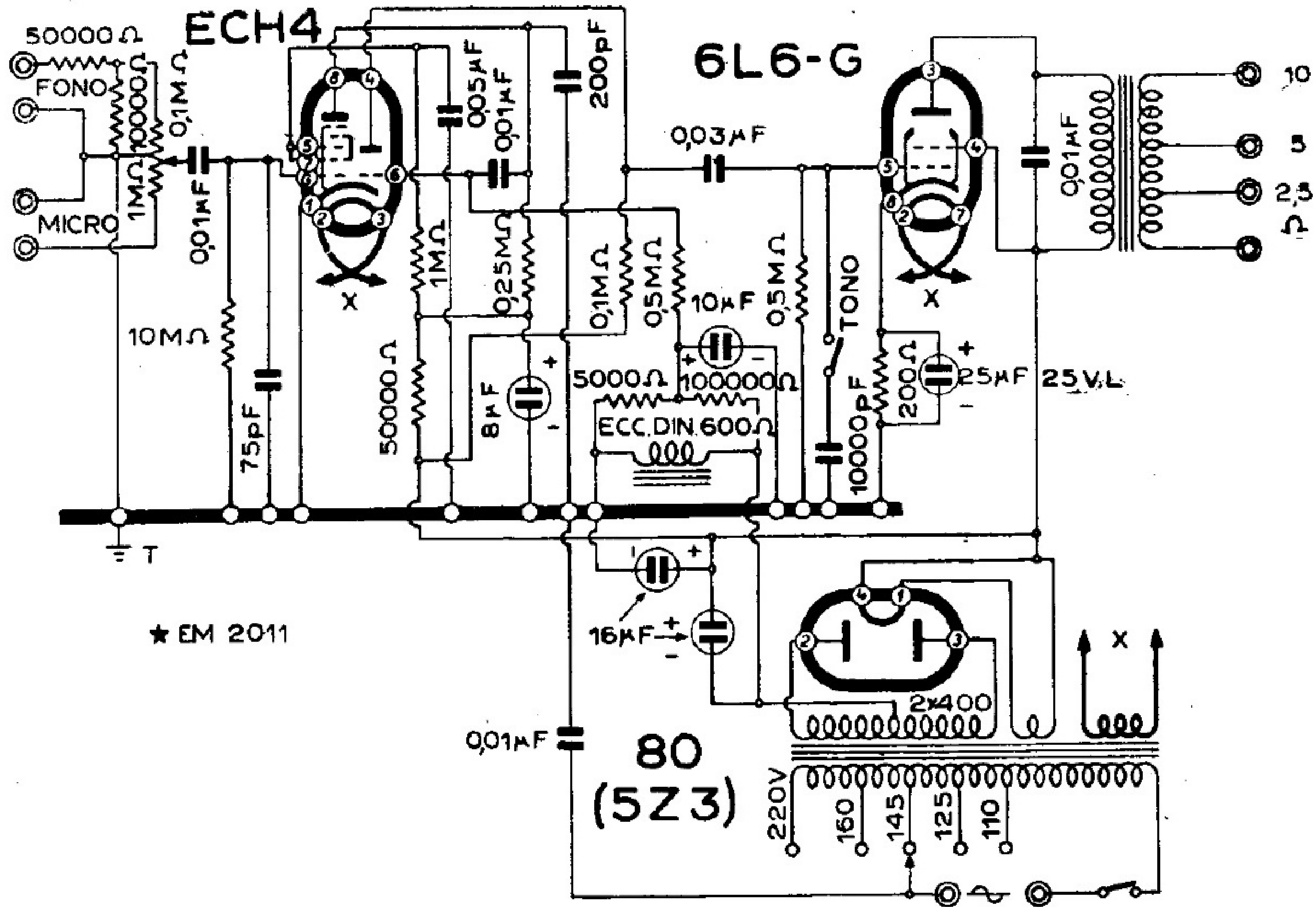
NOVA - AMPLIFICATORE MOD. « 10 W - VICTOR »
