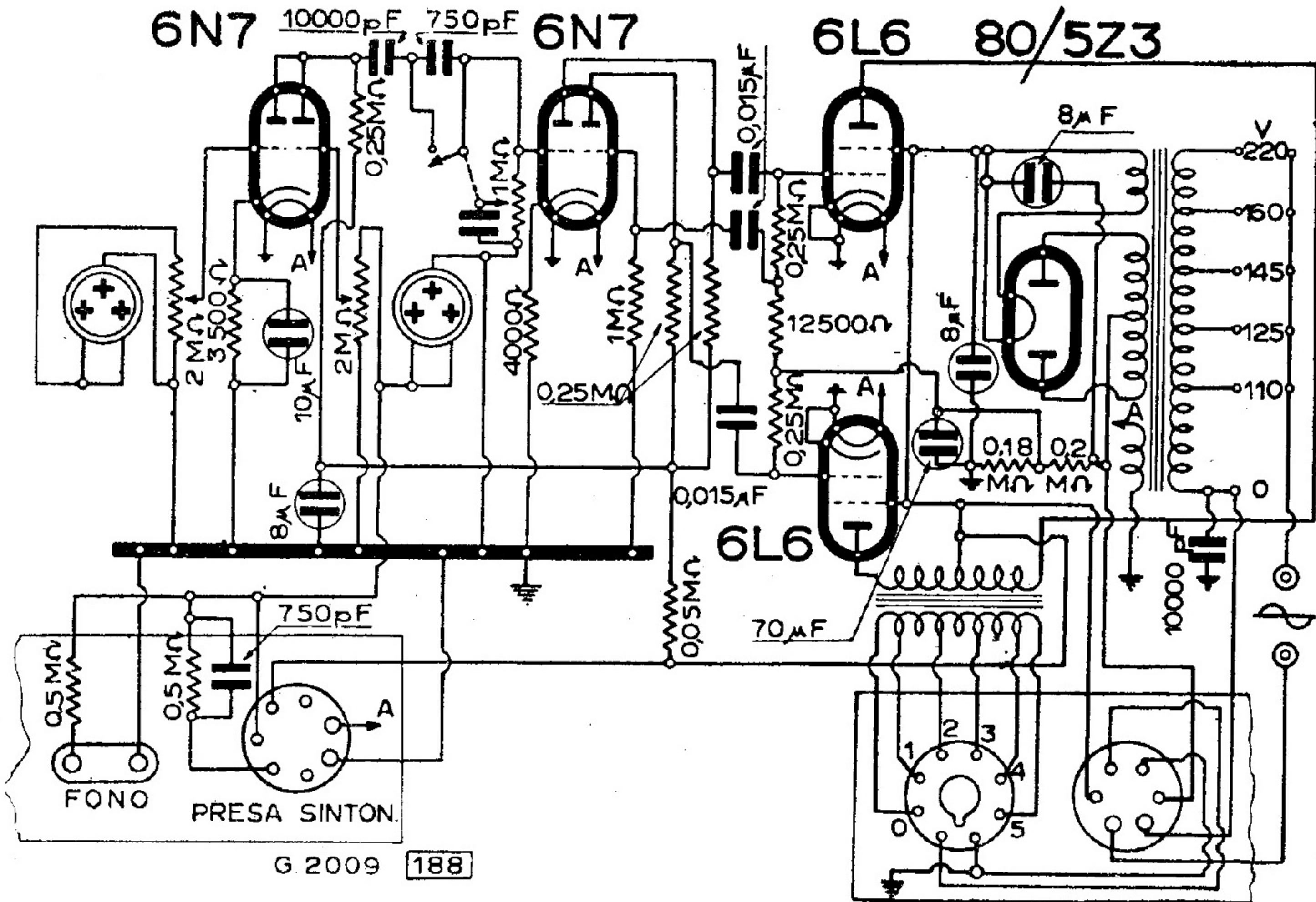
NOVA - AMPLIFICATORE MOD. « 20 W »
