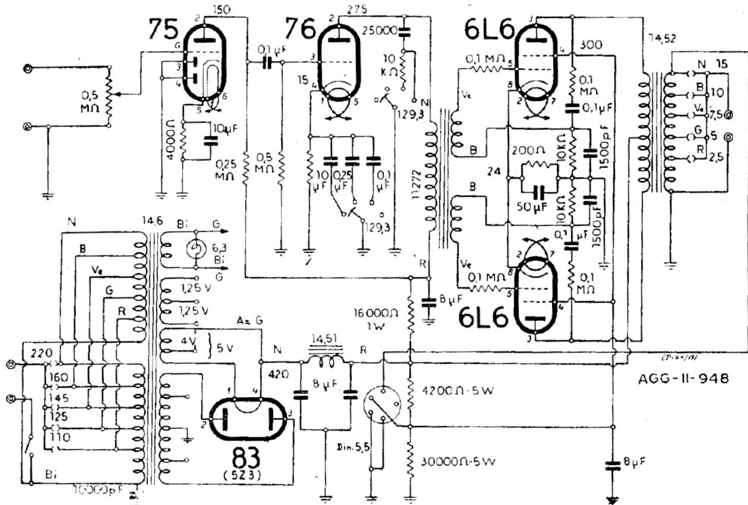
NOVA - AMPLIFICATORE MOD. « 24-30 W » - Nuova Serie
