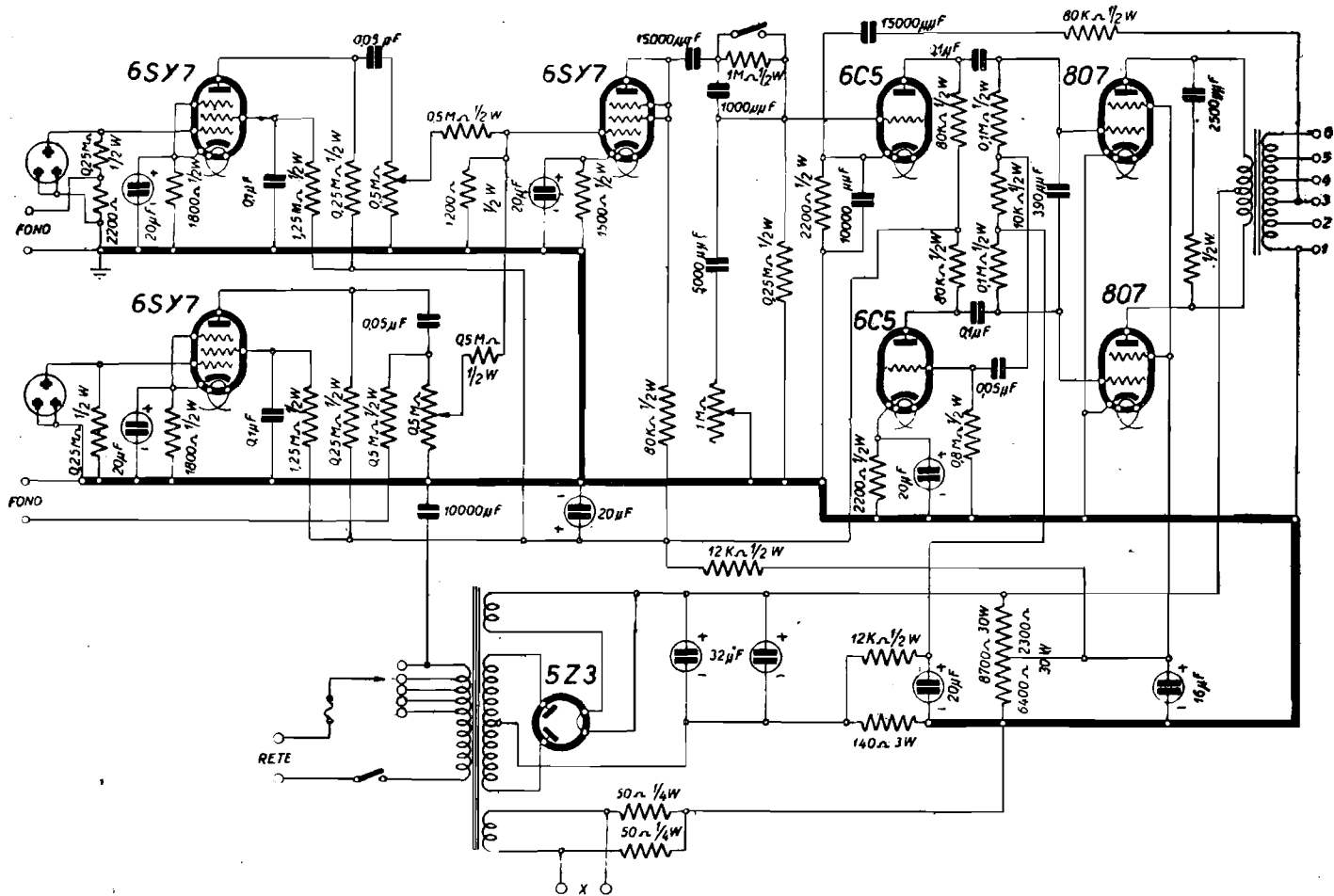
NOVA - Mod. VICTOR 25-30. Potenza da 25 a 30 watt. Impedenze d'uscita comprese tra 0,6 ohm e 250 ohm, secondo combinazione tra i morsetti. Tensioni: 395 V placca 280 V schermo, 24 V catodo delle 807. Il modello 301 è simile, con 6J5 al posto delle 6C5 e 5x4 al posto della 5Z3.
