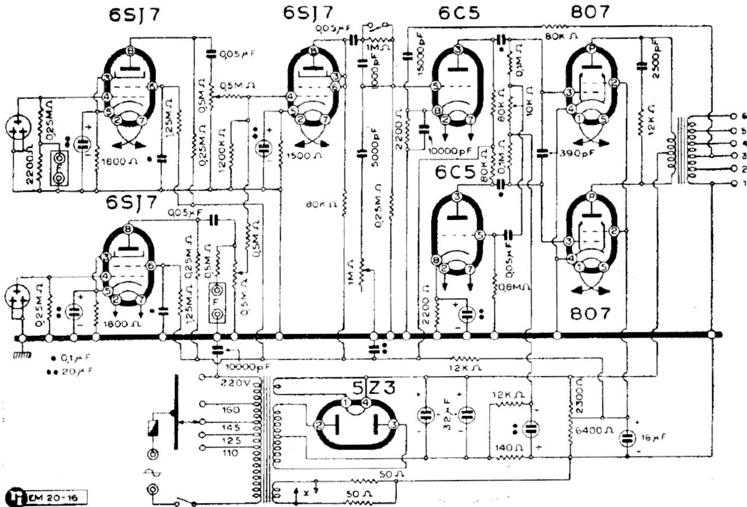
NOVA - AMPLIFICATORE MOD. « 25-30 W - VICTOR »
