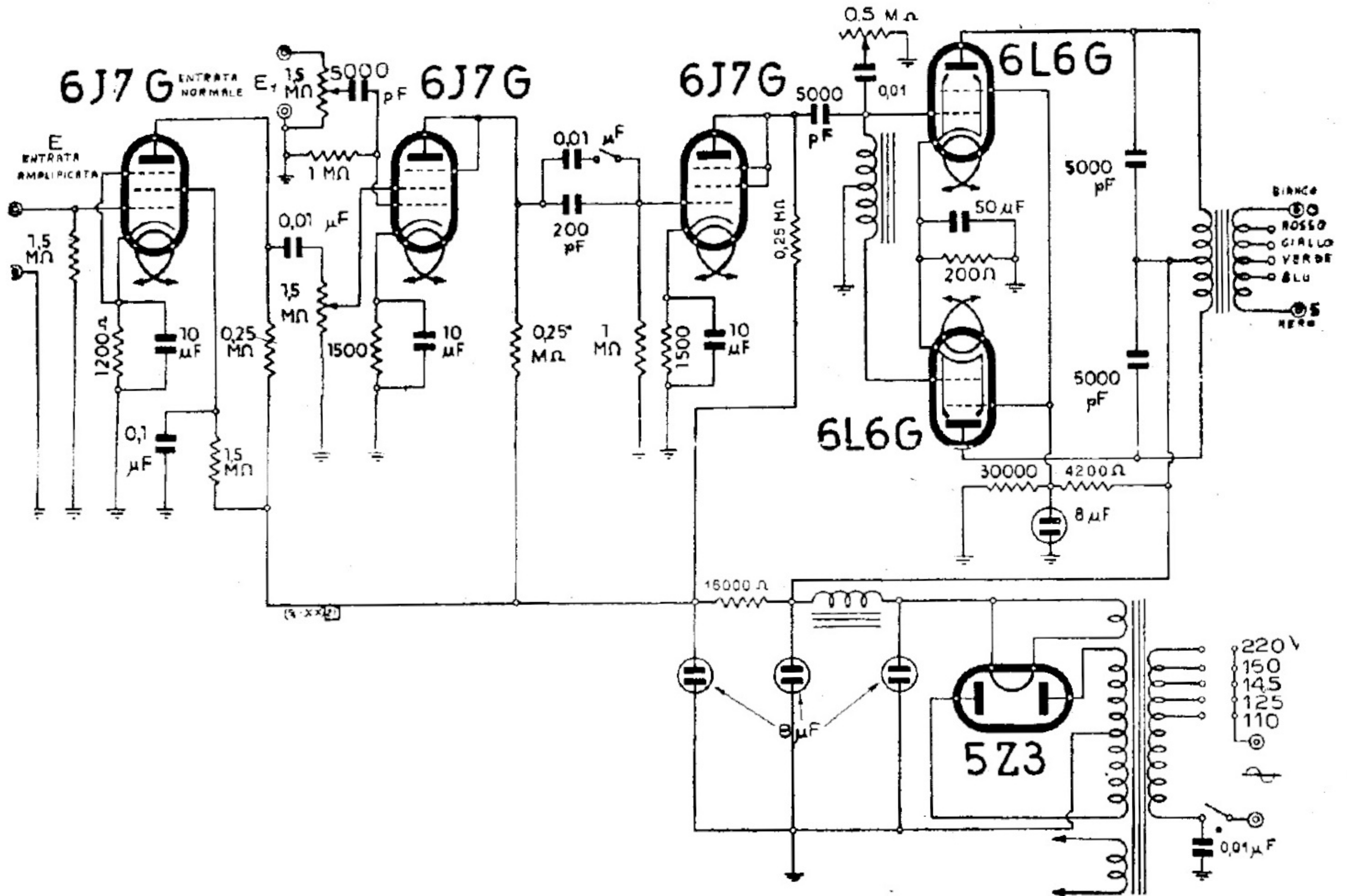
NOVA - AMPLIFICATORE MOD. « 32 W »
