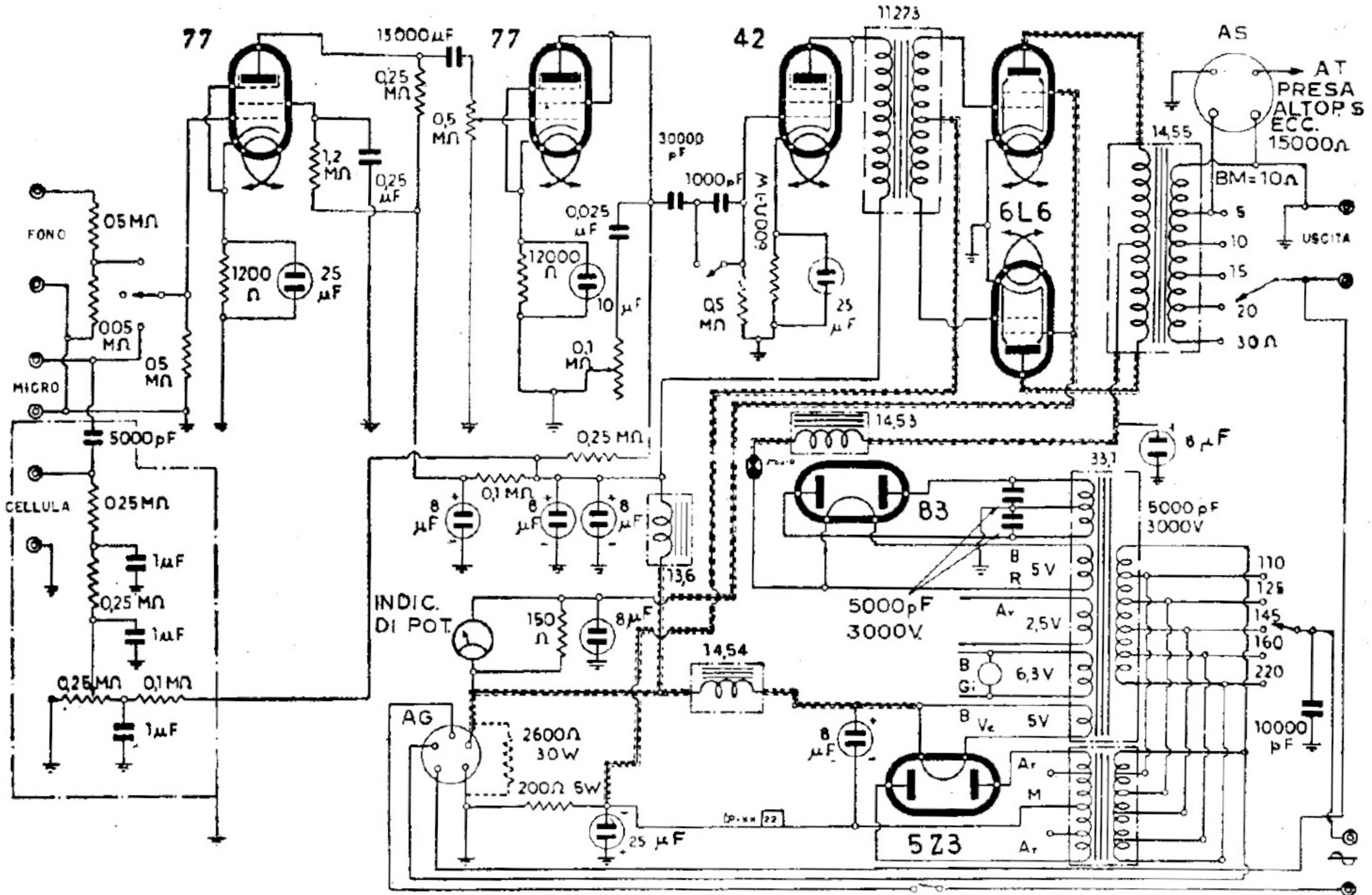
NOVA - AMPLIFICATORE MOD. « 60 W »
