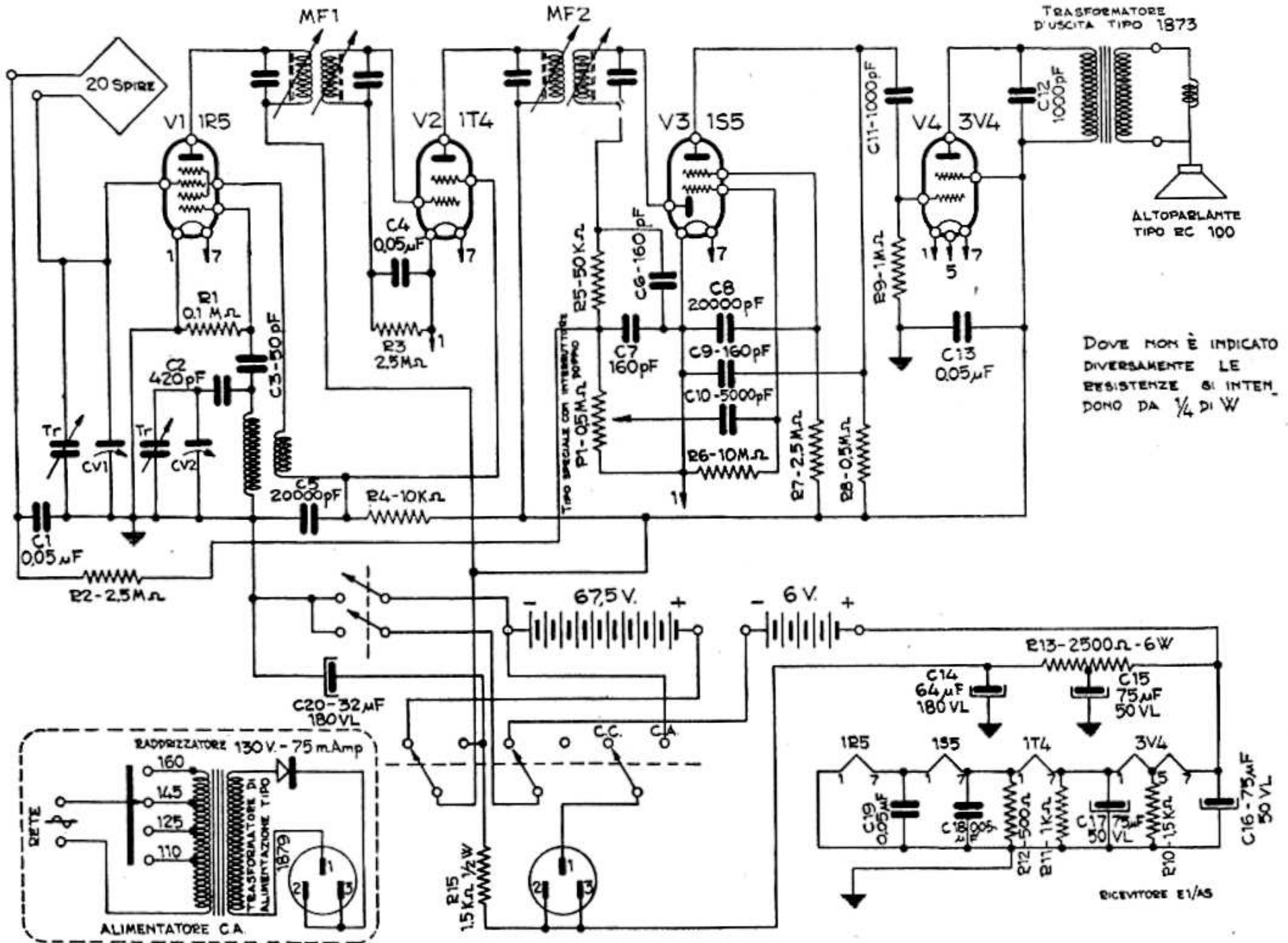
NOVA RADIO - Modd. AS e E1 - Portatile alimentato con pile e adatto per funzionare anche con la tensione alternata dalla rete. Media
