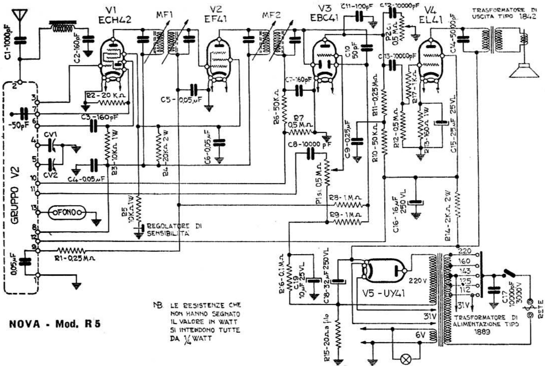
NOVA RADIO - Mod. R5 - Provisto di gruppo alta frequenza mod. V2. Media frequenza 465 kc. Potenza d'uscita 4 watt indistorti.
