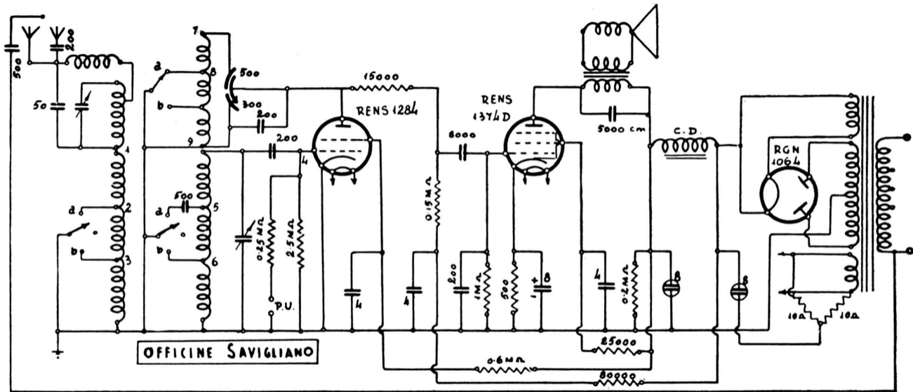
Rivelatrice in reazione seguita da amplificatrice finale. - Tensioni: 410 v. tra filamento 80 e massa, 330 v. all'uscita c. d., 220 v. schermo valvola finale, 200 v. placca rivelatrice, 70 v. schermo rivelatrice.
