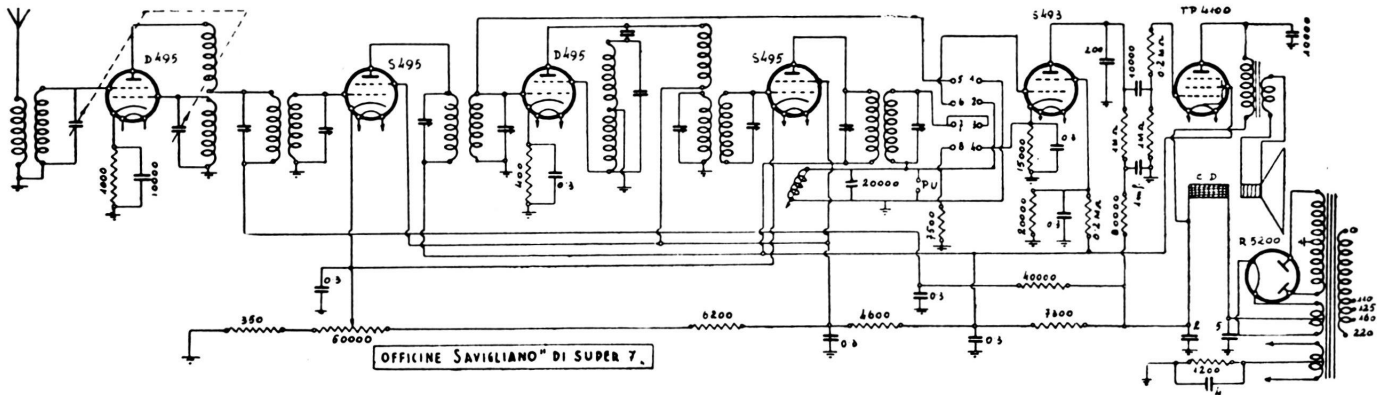
Onde medie. - Circuito a doppia variazione di frequenza con valvole D 495. - Produzione 1933. - Potenza d'uscita: 3 watt.
