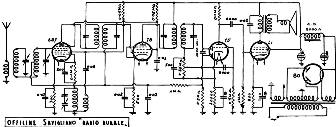
Onde medie. - M. F. 175 kc. - C. A. V. - 6A7 oscill.-modul; 78 amplif. m. f.; 75 demodul.-c.a.v.; 41 finale di potenza. - Potenza d'uscita: 2,5 watt.
