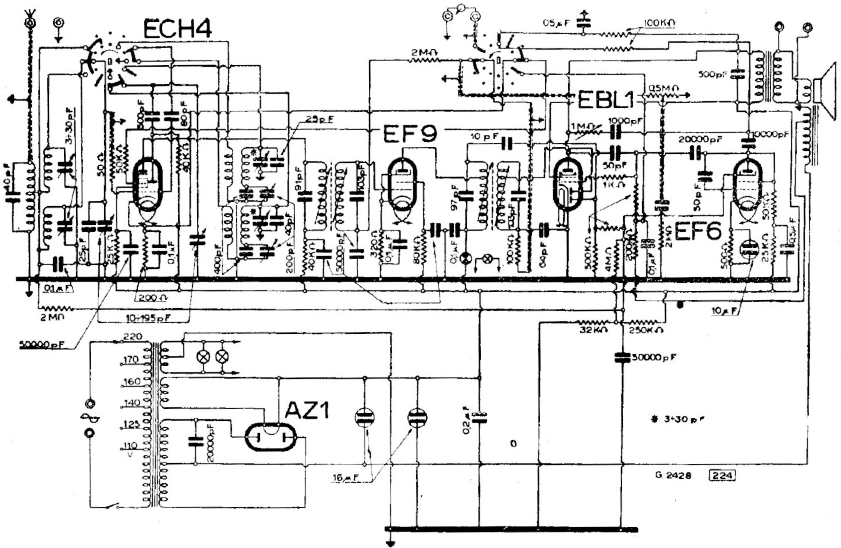
PHILIPS RADIO - MOD. « 478-IV »
