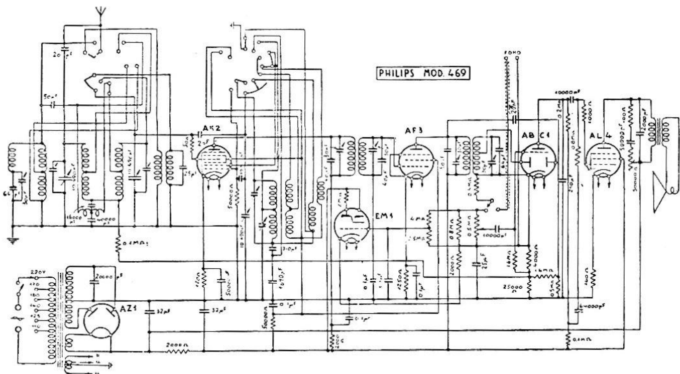
PHILIPS RADIO. — Mod. «469, 777 M e 777 R F». — Produzione 1938-39. — Media frequenza: 468 kHz.
