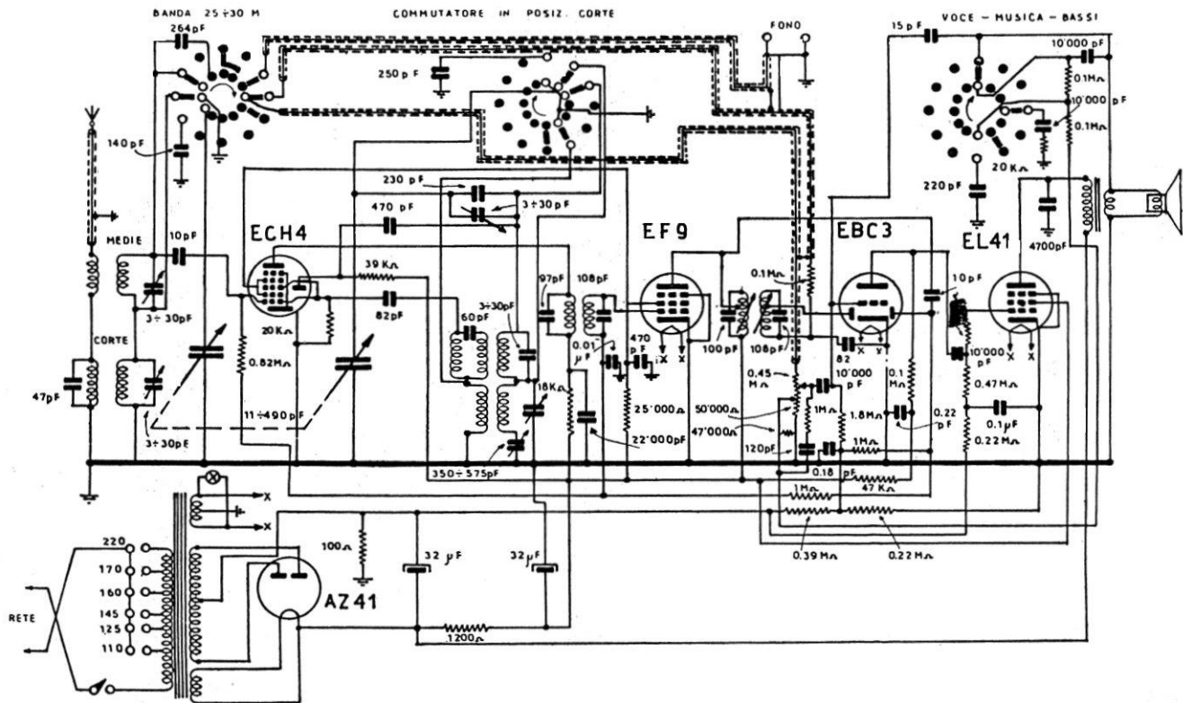
PHILIPS RADIO - Modd. BI 482/A, BI 483/A, BI 490/A e BI 490/A bis - Schema del BI 490A bis. Negli altri modelli le tre ultime valvole sono le seguenti: EF6, EBL1 e AZ1. Media frequenza 468 kc.
