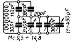
CIRCUITO OSCILLANTE
