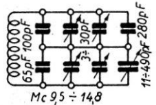
CIRCUITO D'ANTENNA
