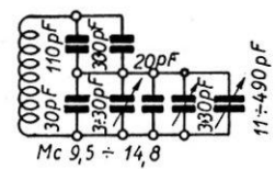
CIRCUITO OSCILLANTE
