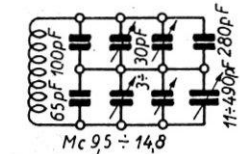
CIRCUITO D'ANTENNA
