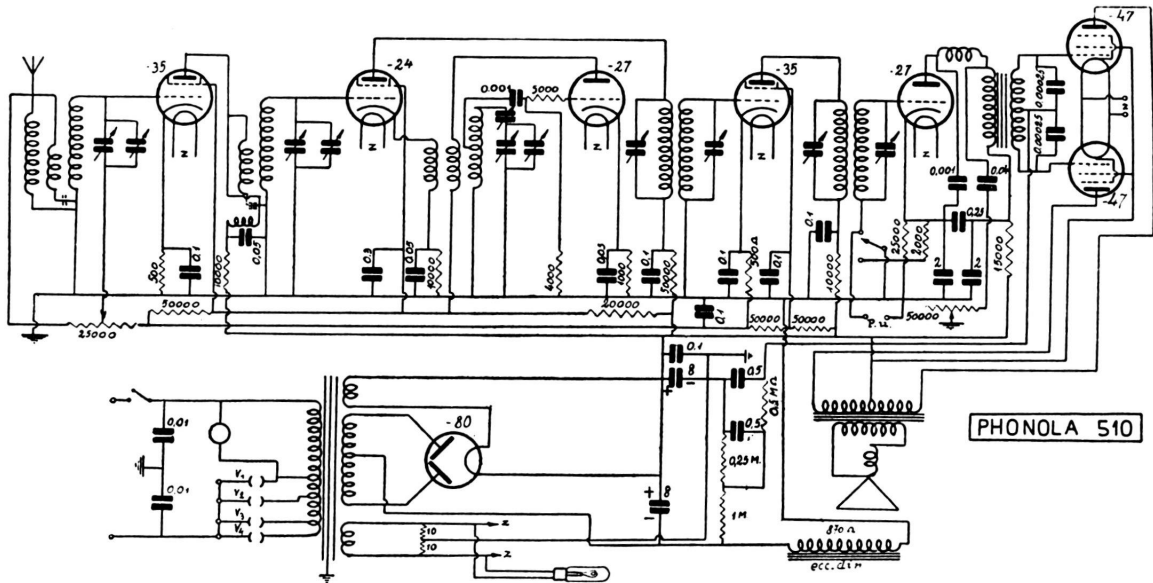
Onde medie. - M. F. 175 kc. - Oscillatrice separata 27. - Controfase di 47. - Potenza d'uscita: 4 watt.
