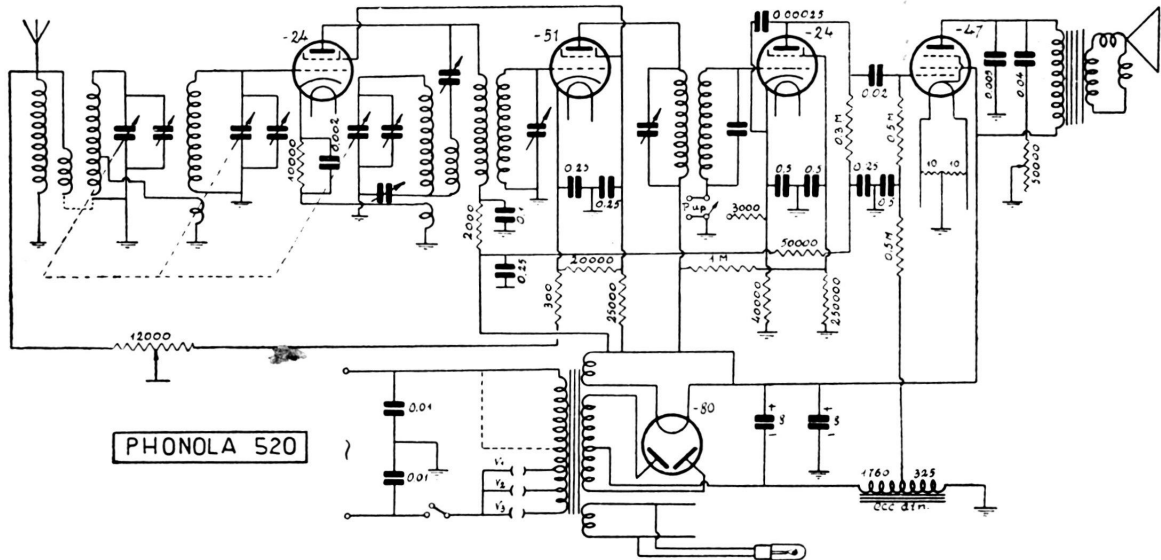
Onde medie. - M. F. 175 kc. - 24 oscillatrice-modulatrice. - 51 amplificatrice m. f. - 24 demodulatrice. - 47 finale. - Potenza d'uscita: 2.5 watt.
