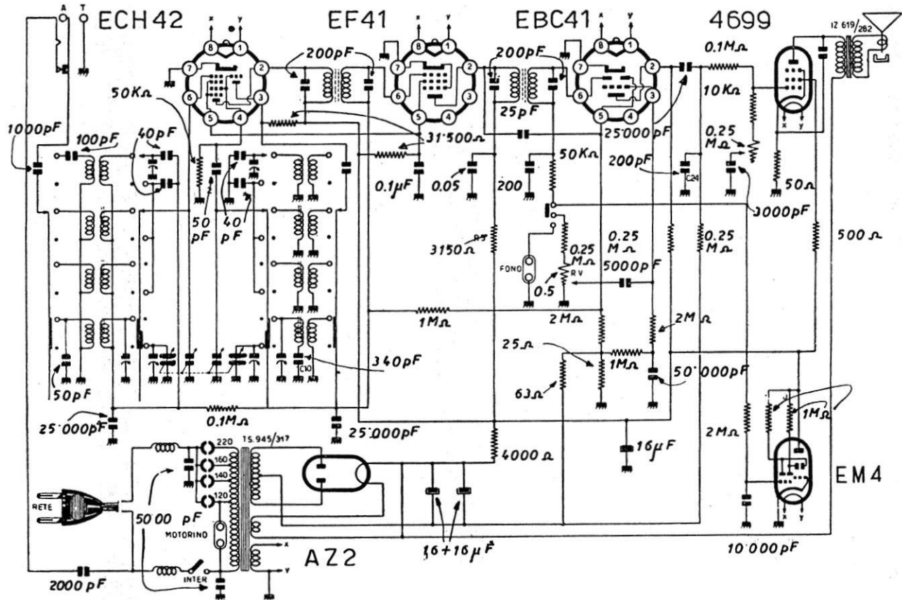
PHONOLA RADIO - Modd. 5512 A/B, 5517 A e 5518 - Medie divise e cinque bande onde corte. 5512 B radiofonografo: 5518 altoparlante M 201. MF a 470 kc. Placca finale 270 V, schermo 250 V. Altre placche 250 V, schermi 90 V. Uscita 6 W.
