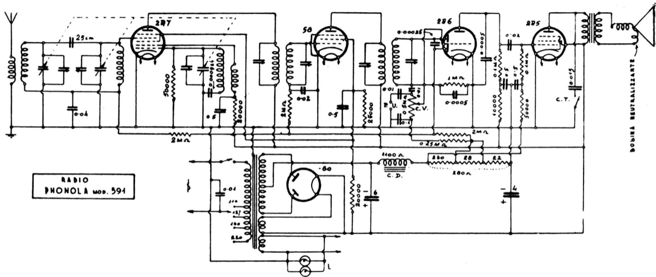
Onde medie. - M. F. 175 kc. - C. A. V. - 2A7 oscill.-modul. con accoppiamento elettronico; 58 amplif. m. f.; 2A6 demodul.-c.a.v.; 2A5 finale di potenza a polarizzazione fissa. - Variatore tono. - Potenza uscita: 3 w.
