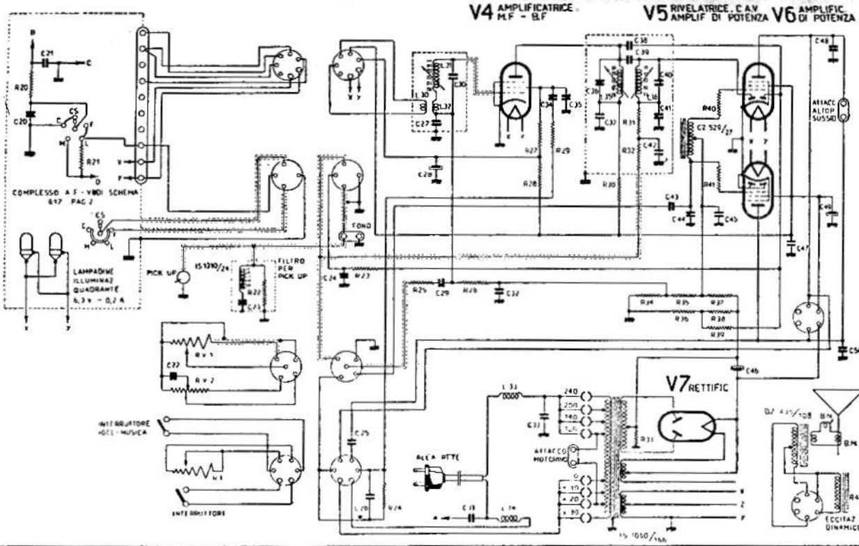
PHONO LA (S. A. FIMI). — Mod. 710. — Compl. MF e BF. (Complesso A. F. quello del mod. 617). — Produzione 1939. Media frequenza: 470 kHz.
