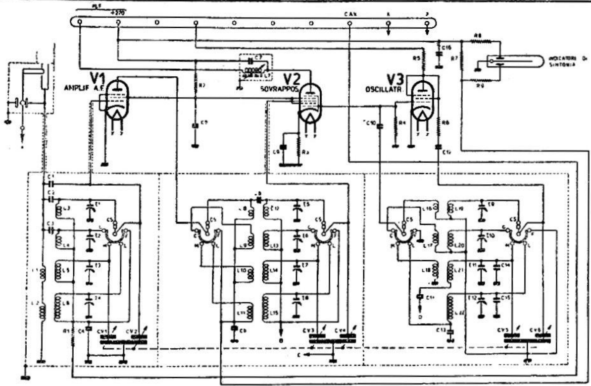
PHONOLA (S A FIMI). — Mod. 617. — Complesso A. F. — Serie ultraconverto. — Produzione 1938-39 — Media frequenza: 470 kH.
